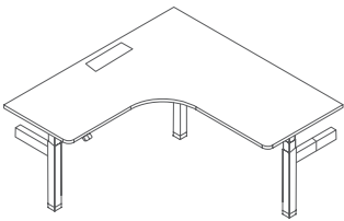
FIT L 形升降桌 1600L * 700W * 1600L * 600W * 750 ~ 1250H 1800L * 700W * 1800L * 600W * 750 ~ 1250H
