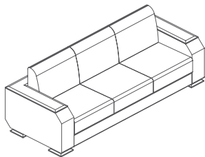
SF-HUADI-1S 1070L*950W*800H SF-HUADI-2S 1690L*950W*800H SF-HUADI-3S 2310L*950W*800H
