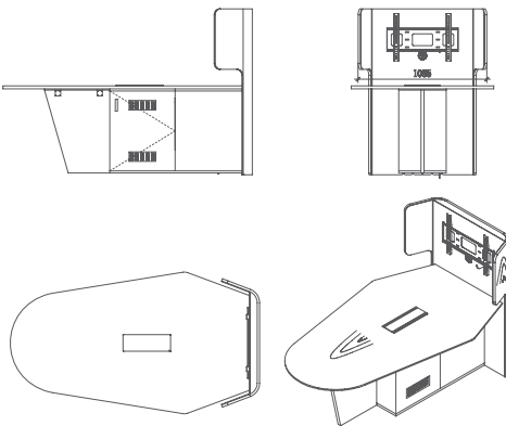
VC-T01 2085L*1200W*1400H 台高 750H
