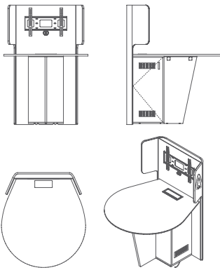
VC-T02 1350L*1200W*1700H 台高 1000H
