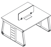
HXOD 双边组合 1200L*1200W*1050H 1400L*1200W*1050H
