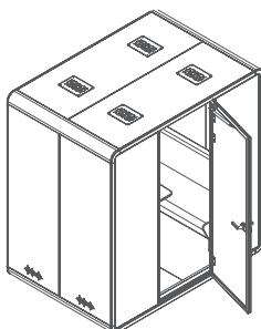
HUSH - I -L01 四人洽谈间 2200L * 1520W * 2300H
