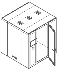
HUSH-XL01 会议间 2200L * 2100W * 2300H
