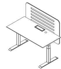
FIT 单人工位 1400L * 700W * 750 ~ 1250H 1600L * 700W * 750 ~ 1250H
