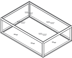
安伯茶几 01 1200L * 820W * 370H
