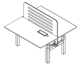
FIT 双人工位 1400L * 1420W * 750 ~ 1250H 1600L * 1420W * 750 ~ 1250H
