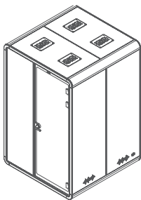
HUSH - I -M01 双人洽谈间 1500L * 1520W * 2300H
