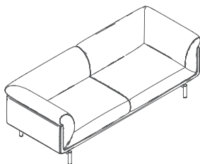
三人位沙发 2150L * 850W * 730H
